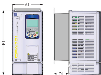
Frame sizes A, B and C with Nema1 kit Tamaños A, B y C con kit Nema1 Mecânicas A, B e C com kit Nema1
