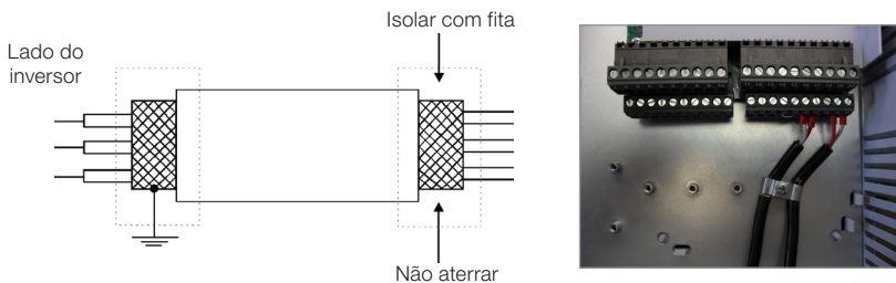
(b) Exemplo de ligação da blindagem ao terra
