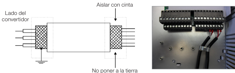
(b) Ejemplo de conexión del blindaje al punto de tierra
