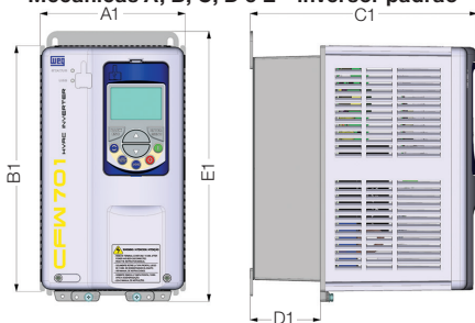
Frame sizes A, B, C, D and E – standard inverter Tamaños A, B, C, D y E – convertidor estándar Mecânicas A, B, C, D e E – inversor padrão
