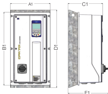
Frame sizes B and C with degree of protection IP54 Tamaños B y C con grado de protección IP54 Mecânicas B e C com grau de proteção IP54
