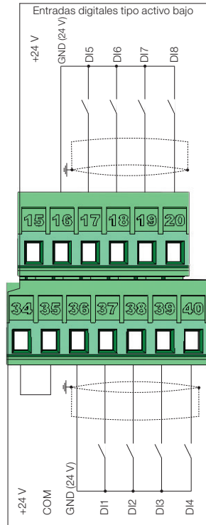
(c) Entradas digitales tipo activo bajo
